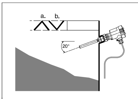
Abb. 2: Horizontaler Einbau
