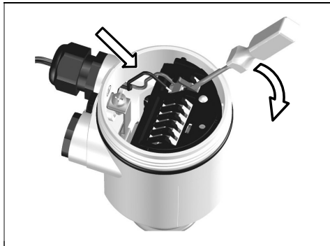
Abb. 3: Anschlussschritte 5 und 6
