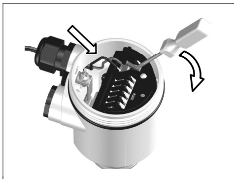
Fig. 19: Étapes de raccordement 5 et 6
