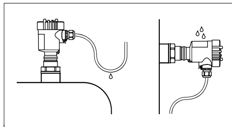
Fig. 25: Medidas contra la entrada de humedad
