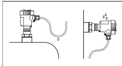
Abb. 1: Maßnahmen gegen das Eindringen von Feuchtigkeit
