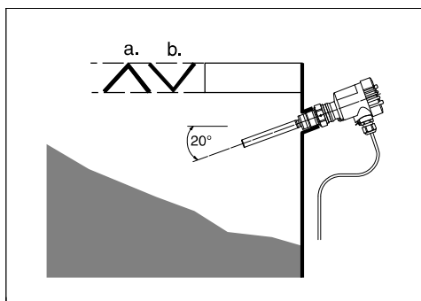
Fig. 18: Montage horizontal
