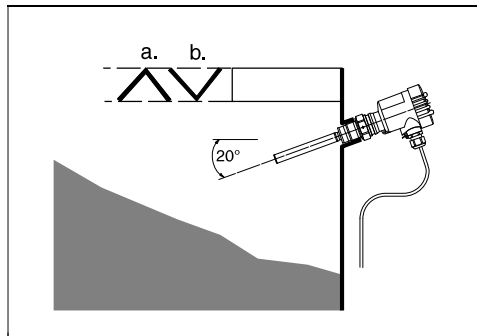
Fig. 26: Montaje horizontal
